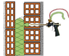
Inyección de aislante
