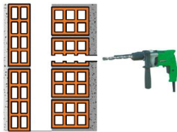
Perforaciones hasta la cámara
